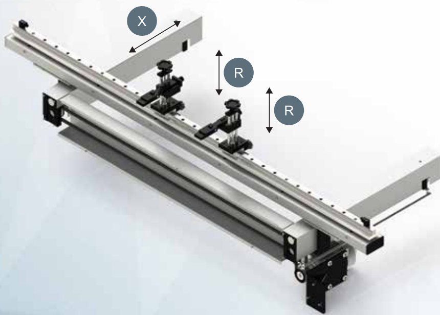
Стандартный задний упор X ось ЧПУ R ось ручная
